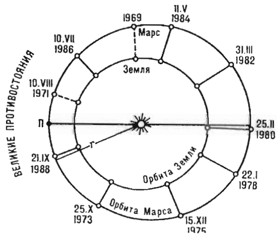
Противостояния Марса; П — перигелий орбиты Марса, великие противостояния — 1971, 1986, 1988.
